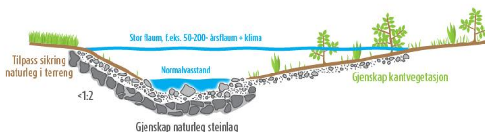
Figur 7-1 Skisse for opning av bekk. NVE, basert på ei teikning frå NORCE.
