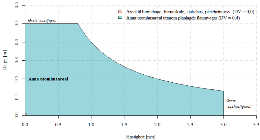
Figur 4-3 NVEs tilråding – fare for menneske på utomhusareal, NVE.
